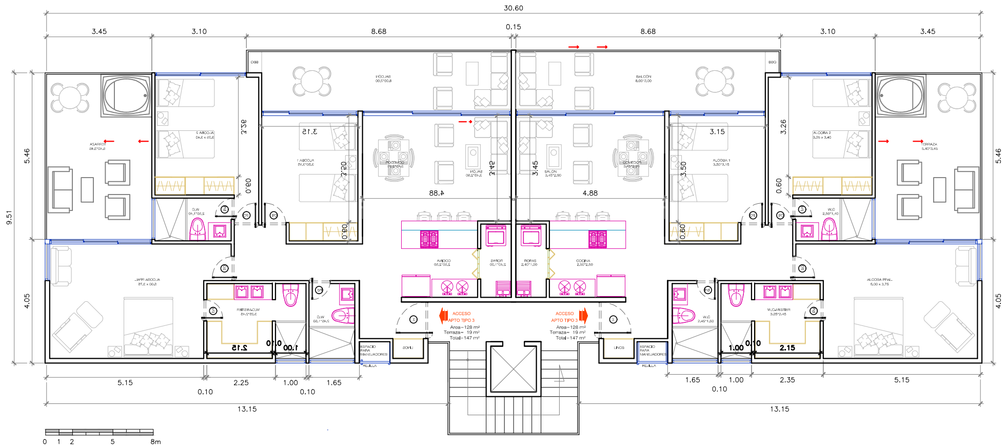
GRAND VIEW PLANTA TIPICA APTOS. NIVEL 4 ESC 1 :100
